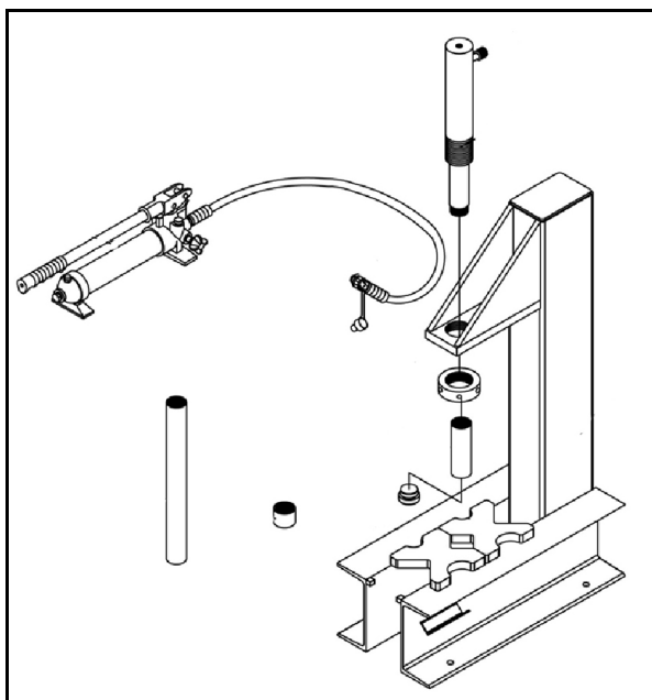
Obr. 6: Montáž dílů
