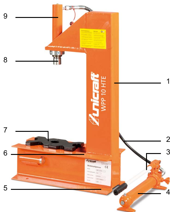
Obr. 4: Popis stroje
