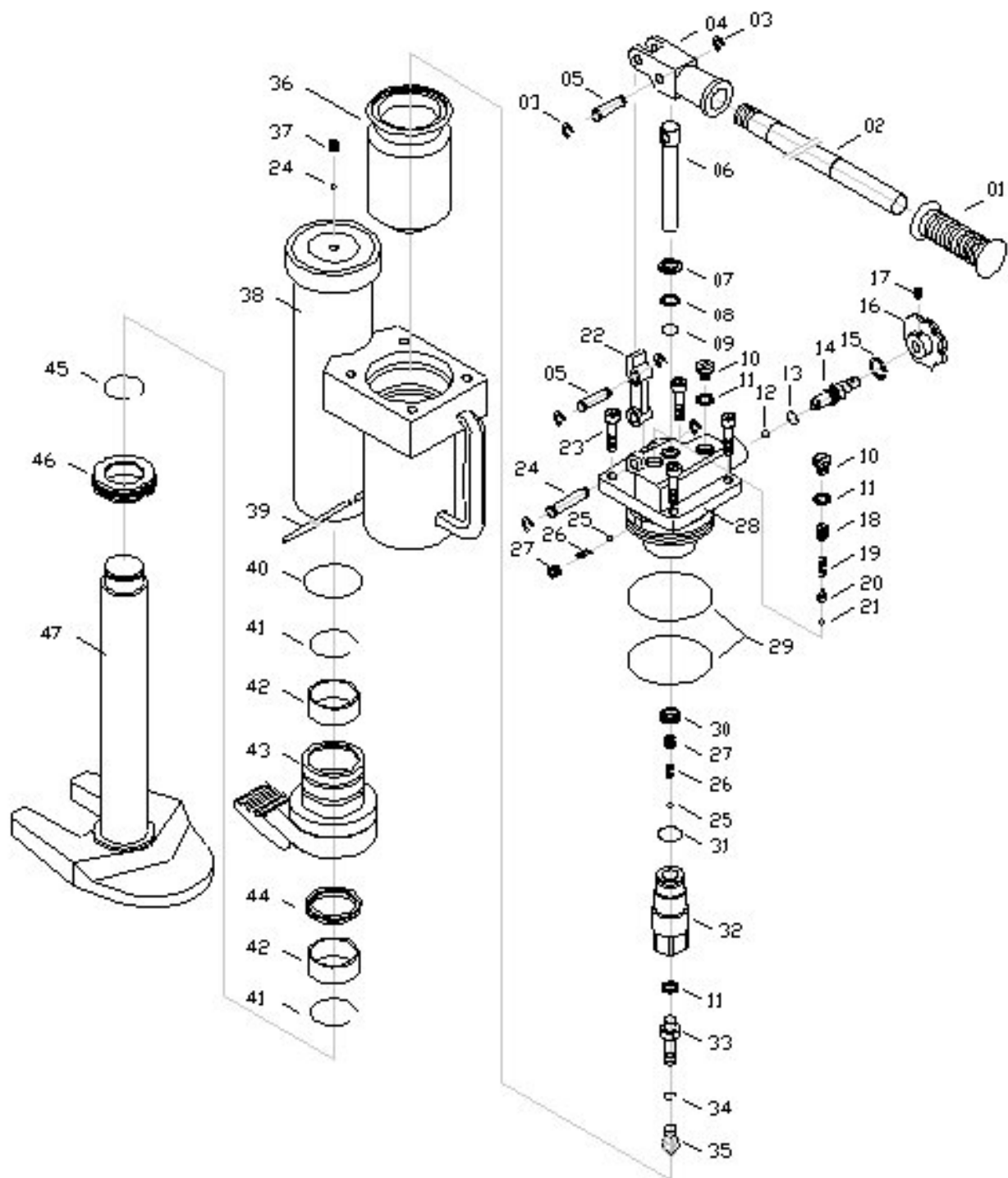
Abb. 1: Ersatzteilzeichnung HMH 5 & HMH 10 / Spare parts drawing HMH 5 & HMH 10
