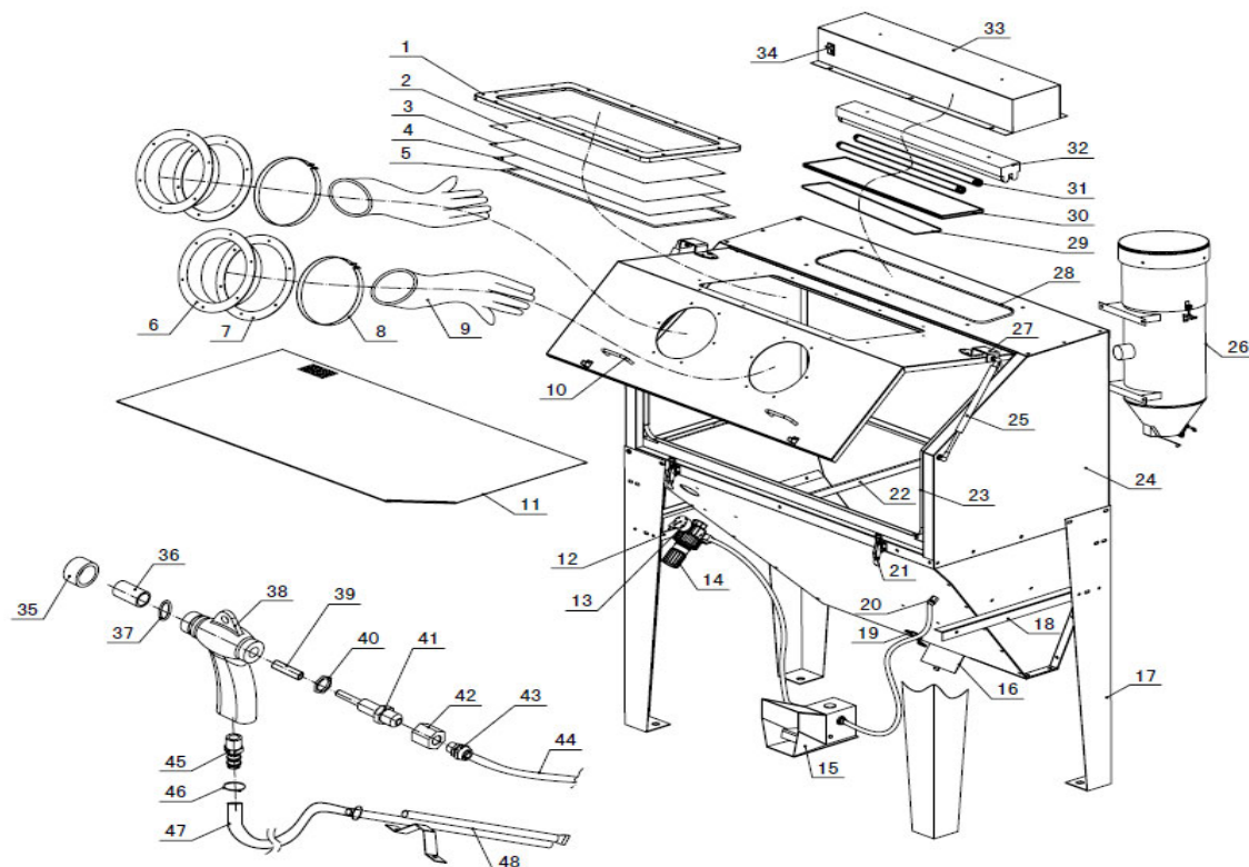
Obr. 6: Rozpadové schéma SSK 3.1
