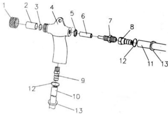
Obr. 4: Pískovací pistole
