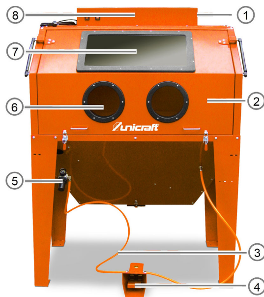
Obr. 2: Pískovací box SSK 3.1
