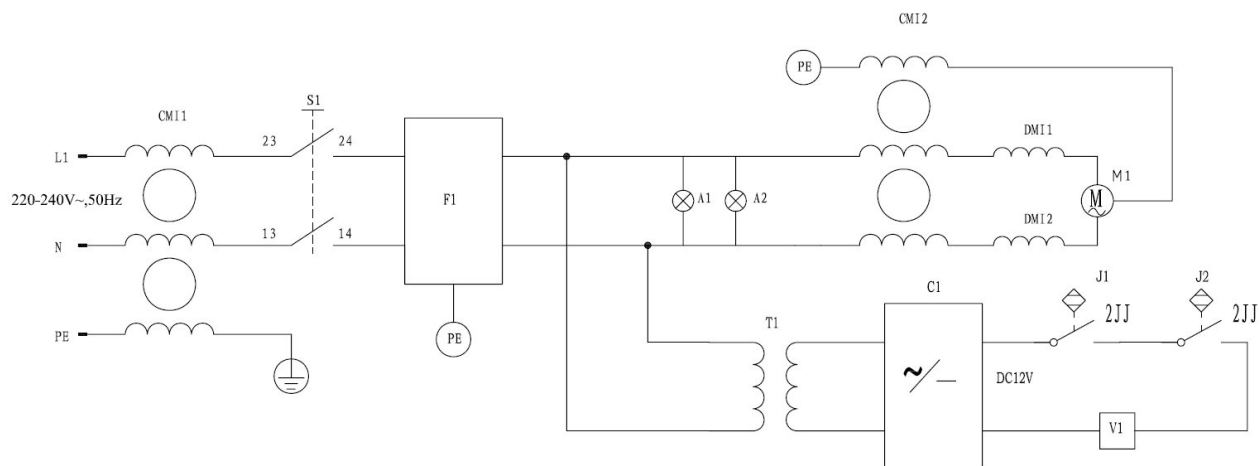
Obr. 7: Schéma zapojení
